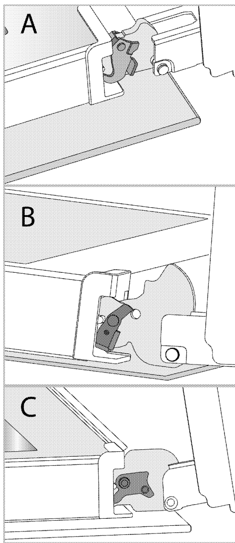
Закључване на панти - отворено положение
