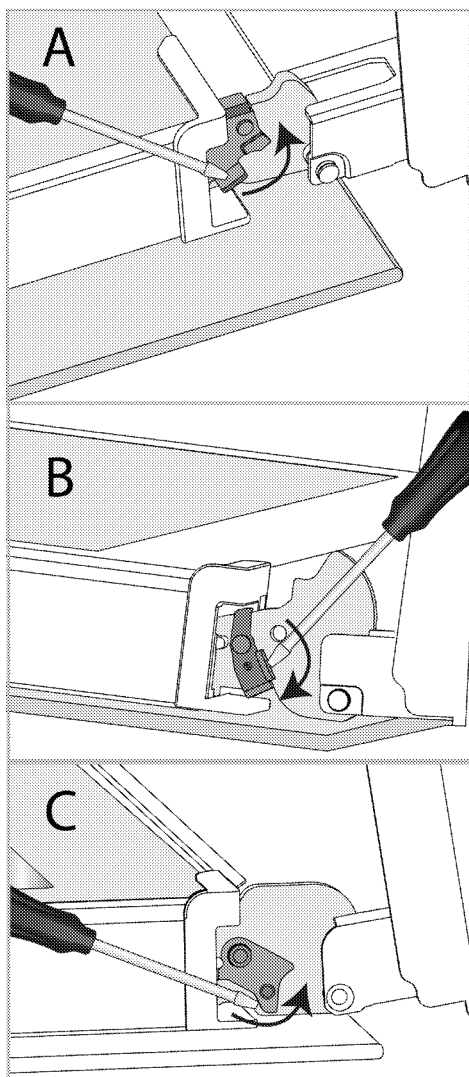
Закључване на панти - затворено положение
