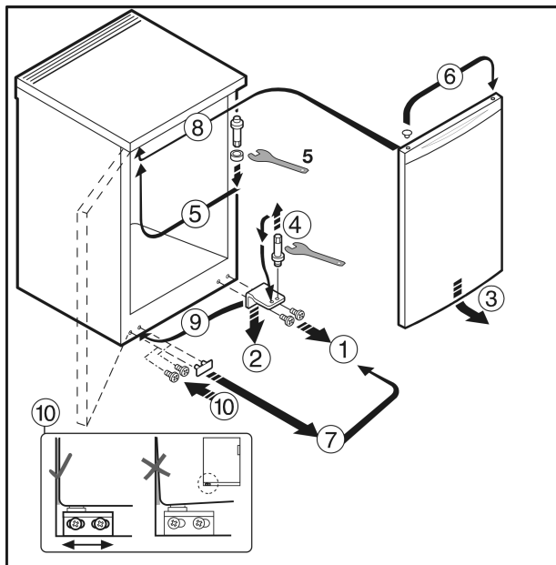
Fig. 5 при уреди без дръжка на вратата*
